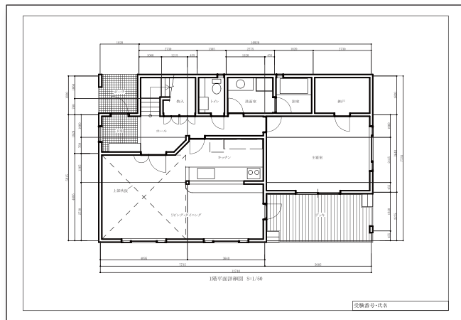
1 階平面詳細図(S=1/50)
